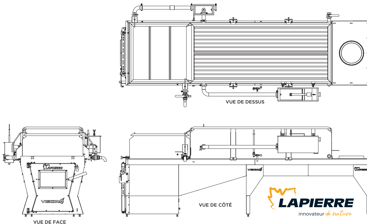
ILLUSTRATION 3 | Illustration type d'un évaporateur VISION 6 pattes
