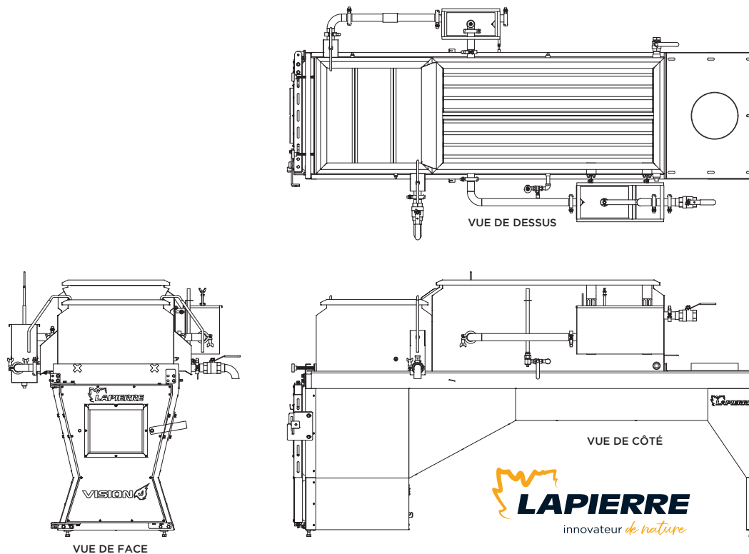
ILLUSTRATION 2 | Illustration type d'un évaporateur VISION 4 pattes
