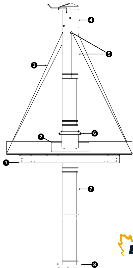
ILLUSTRATION 1 | Cheminée type d'un évaporateur
